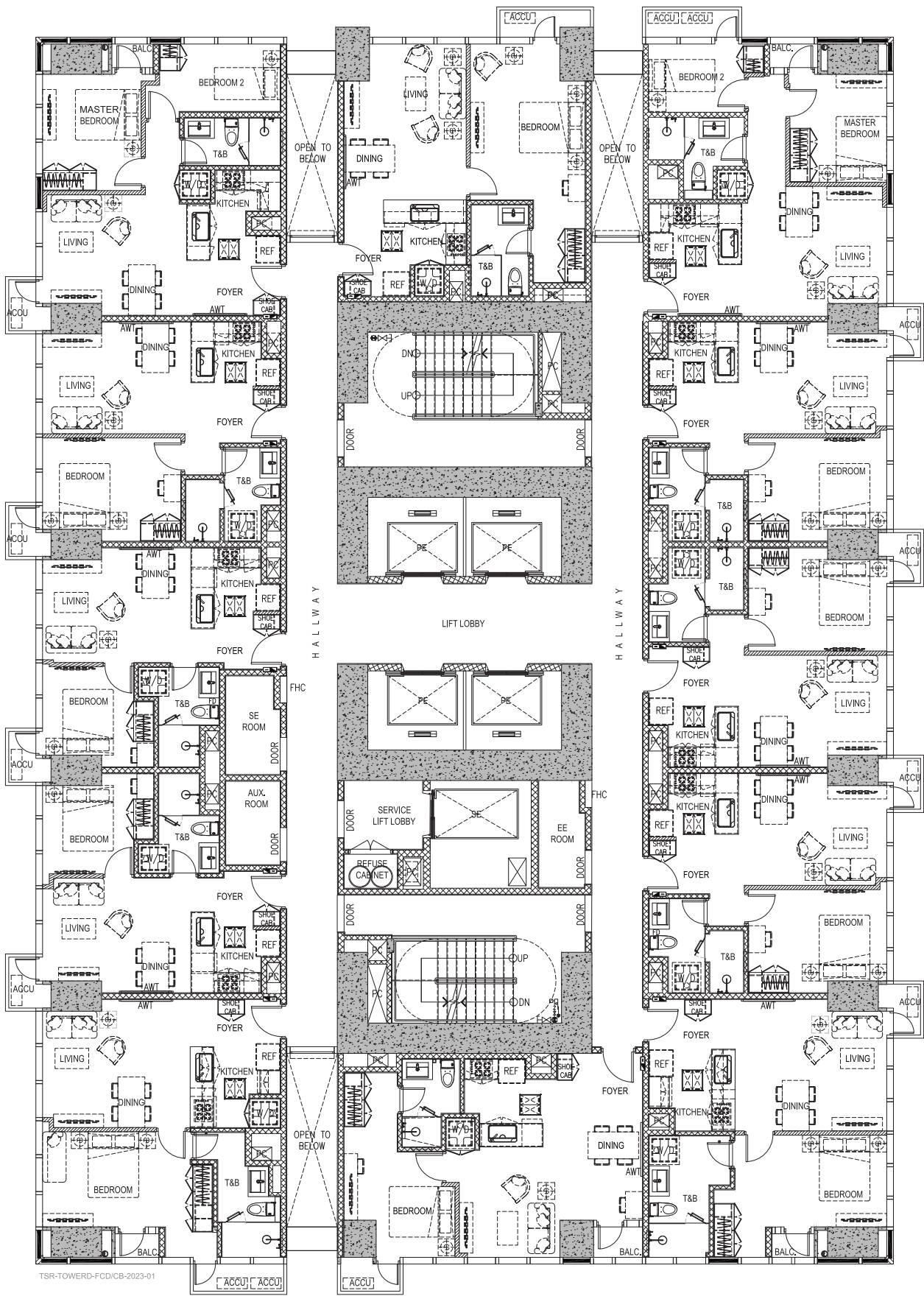
A 1BR SUITE 60 sqm
